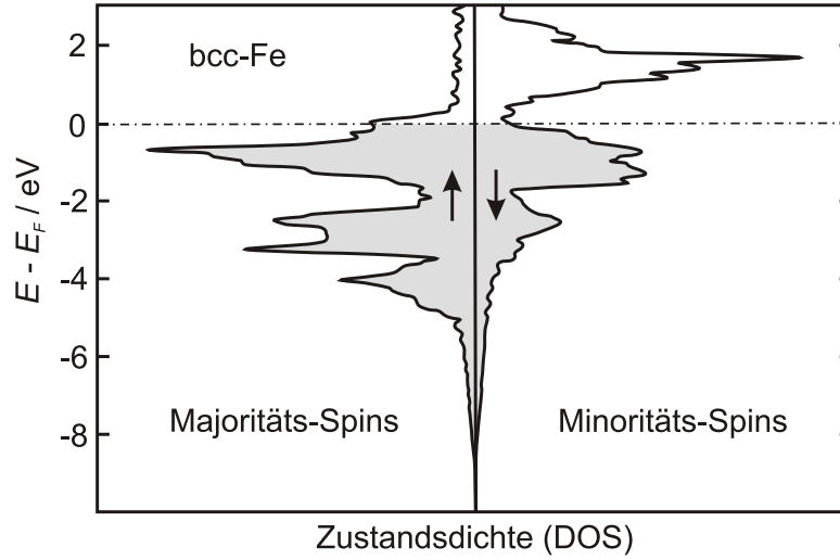
Abbildung 3.8: Mit LDA-ASW berechnete Zustandsdichte der Majoritäts- und Minoritäts-Ladungsträger von ferromagnetischem Eisen mit einer bcc Kristallstruktur. Die Form der spin-up(↑) und spin-down(↓) DOS ist in erster Näherung identisch. Beide DOS sind jedoch energetisch gegen einander verschoben, was in einem Überschuss an Majoritäts-Spins resultiert [43].
