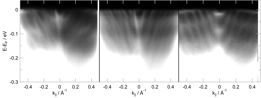
Abbildung A.8: ARPES-Datensätze (original, h\nu = 21.2 eV) von 12, 14 und 21 ML Ni/W(110). Die Aufspaltung der leichten QWS wird mit zunehmender Schichtdicke kleiner, bei 21 ML ist keine Aufspaltung mehr erkennbar.
