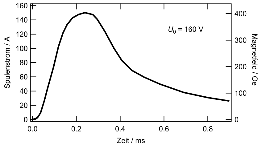
Abbildung 6.10: Durch eine Kondensatorentladung erzeugter Spulenstrom durch das zur Magnetisierung der Ni-Filme benutzte Helmholtzspulenpaar als Funktion der Zeit. Gezeigt ist eine Eichmessung bei einer Ausgangs- bzw. Kondensatorspannung von U_0 = 160 V. Zur Probenmagnetisierung wurden höhere Spannungen von ca. 260 V verwendet. Die rechte Achse gibt das dem Spulenstrom entsprechende Magnetfeld an der Probenposition an.
