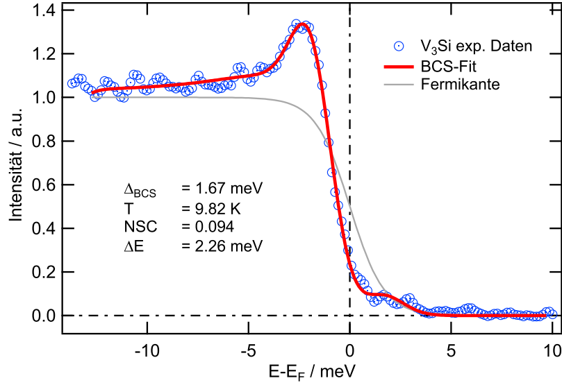
Abbildung 2.3: UPS-Spektrum einer supraleitenden V_3Si -Probe. Gezeigt sind experimentelle Daten ( E_{pass} = 2 eV, Spaltbreite 0.1 mm, fixed-mode ) zusammen mit einem auflösungsverbreiterten BCS-Fit. Zum Vergleich dazu ist eine Fermikante bei der ermittelten Temperatur von 9.82 K geplottet.
