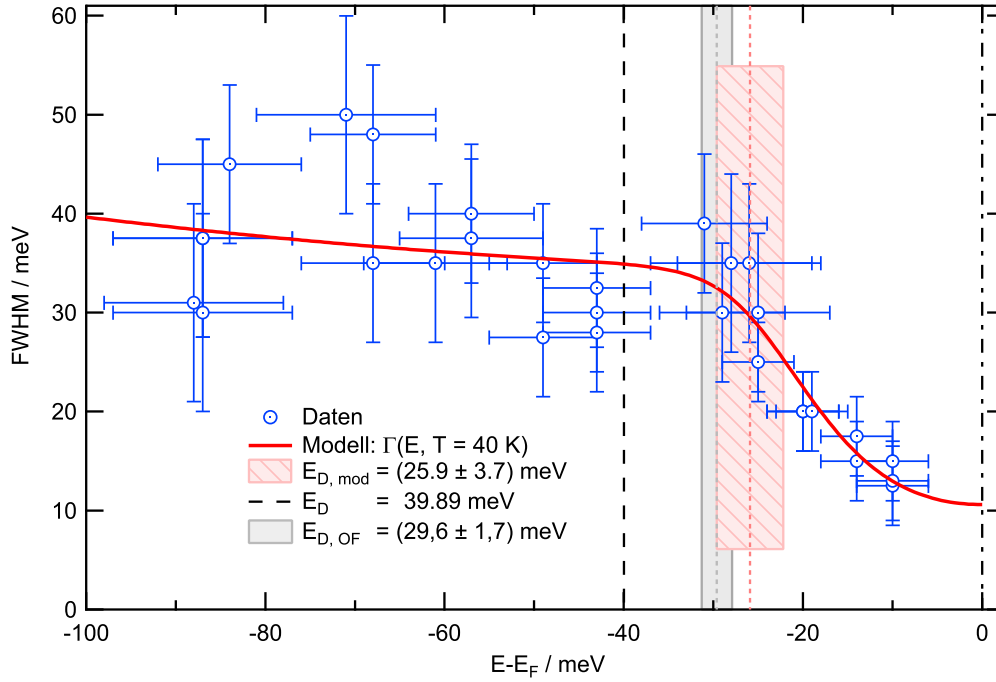
Abbildung 5.5: Linienbreiten der QWS am \bar{\Gamma} -Punkt von Fe/W(110) als Funktion der Energie. Die Datenpunkte ergeben sich aus Messungen von mehreren Schichtdicken. An die Daten wurde das Modell (5.1) für eine Temperatur von 40 K angepasst (rot). Die daraus ermittelte Debye-Energie E_D = (25.9 \pm 3.7) \text{ meV} ist hellrot schraffiert hinterlegt. Ebenfalls eingezeichnet wurden die Debye-Energie von Eisen ( E_D = 39.89 \text{ meV} [122], gestrichelte Linie) sowie die Oberflächen-Debye-Energie von 1 ML Fe/Cu(111) ( E_{D, \text{OF}} = (29.6 \pm 1.7) \text{ meV} [123], grau hinterlegt).
