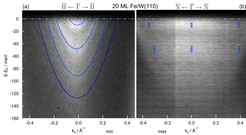
Abbildung A.6: ARPES-Daten von 20 ML Fe/W(110) in (a) \bar{\Gamma}\bar{H} - und (b) \bar{\Gamma}\bar{N} -Richtung.
