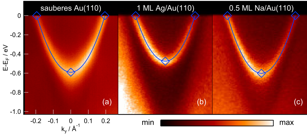
Abbildung 4.11: Vergleich zwischen sauberem, unrekonstruiertem Au(110), 1 ML Ag/Au(110) und 0.5 ML Na/Au(110). Die blauen Linien repräsentieren die Anpassung einer parabolischen Dispersion an die Daten anhand der Stützstellen k_F und E_0
