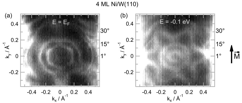
Abbildung A.9: 4 ML Ni/W(110): (a) Fermifläche \mathcal{I}(k_x, k_y)_{E=E_F} , (b) ESM bei -0.1 eV \mathcal{I}(k_x, k_y)_{E=-0.1 \text{ eV}} . Der Ni-Film ist entlang der einfachen Achse \overline{\Gamma K} = k_y magnetisiert.
