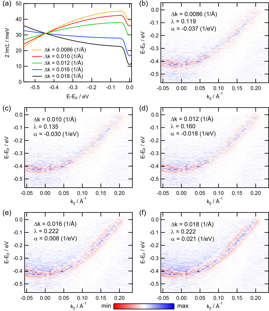
Abbildung A.4: (a) Vergleich der Form von 2 \text{Im}\Sigma(E) aus Anpassungen mit verschiedenen k -Auflösungen \Delta k . Der kleinste Wert ( \Delta k = 0.0086 \text{ Å}^{-1} ) ergibt sich aus einer Anpassung mit \Delta k als freiem Fitparameter. Die funktionelle Form von \text{Im}\Sigma(E) entspricht \text{Im}\Sigma_{\text{e-e}} + \text{Im}\Sigma_{\text{e-ph}} + \text{Im}\Sigma_{\text{e-i}} nach Gleichung (A.2) bzw. (A.3). (b)-(f) zeigen farbcodierte Darstellungen der Residuen zu den Anpassungen aus (a) mit den angepassten Kopplungsparametern für \text{Im}\Sigma_{\text{e-ph}} ( \lambda ) und \text{Im}\Sigma_{\text{e-e}} ( \alpha ). Die Debye-Energie wurde mit \hbar\omega_D = 27 \text{ meV} fest gehalten.
