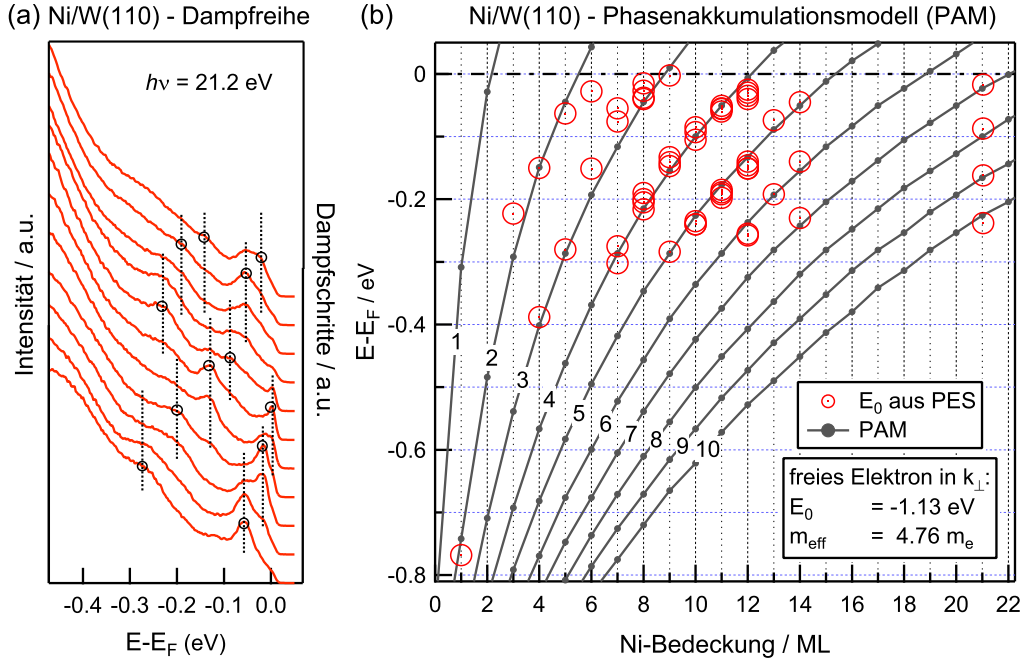
Abbildung 6.9: (a) Bestimmung der QWS-Bindungsenergien einer Dampfreihe von Ni/W(110) aus EDCs ( h\nu = 21.2 eV) bei \bar{\Gamma} . Kreise mit dazu gehörigen gestrichelten Linien markieren die ermittelten QWS. (b) Anpassung eines PAM an alle in dieser Arbeit ermittelten QWS-Bindungsenergien bei \bar{\Gamma} . Als k_{\perp} -Dispersion wurde ein quasi-freies Elektron angenommen. Aus der Anpassung ergeben sich die Parameter E_0 = -1.13 eV und m_{\text{eff}} = 4.76 m_e . Die QWS-Äste sind von 1-10 nummeriert.
