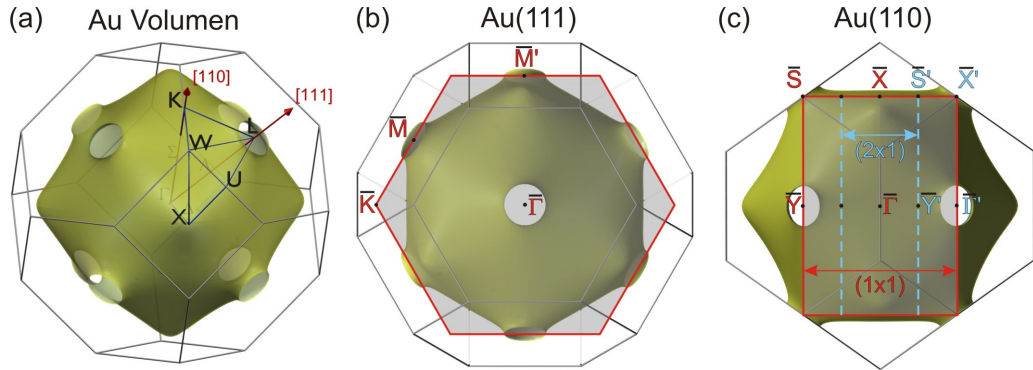
Abbildung 4.1: Dreidimensionale Brillouinzone mit der Fermifläche von Gold [71] aus verschiedenen Blickwinkeln mit eingezeichneten Hochsymmetriepunkten. Die Projektion der in (a) gezeigten Volumenbrillouinzone in eine Richtung resultiert in der entsprechenden Oberflächenbrillouinzone (SBZ) (rot), hier gezeigt für (b) Au(111) und (c) Au(110).
