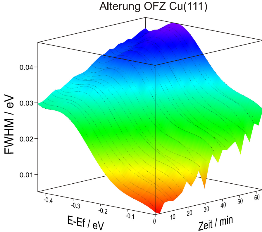
Abbildung A.3: Entwicklung der FWHM ( 2\Im\Sigma ) des OFZ von Cu(111) mit der Messzeit bei einer Probertemperatur von T \approx 70 K. Die prinzipiell lineare Zunahme der Linienbreite mit der Zeit ist für alle Energien erkennbar. Die Steigung \Delta\Gamma des linearen Verlaufs ist jedoch von der Energie abhängig und mit \Delta\Gamma_{E_F} = 0.31 \frac{\text{meV}}{\text{min}} bei E_F größer als \Delta\Gamma_{E_0} = 0.23 \frac{\text{meV}}{\text{min}} bei E_0 = -430 meV.
