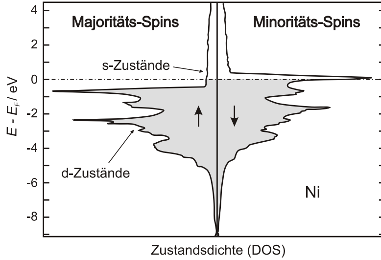
Abbildung 3.9: Berechnete Zustandsdichte der Majoritäts- und Minoritäts-Spins von ferromagnetischem Nickel. Die Majoritäts-d-Zustände liegen komplett unterhalb von E_F während die Minoritätszustände an der oberen Kante von der Fermienergie geschnitten werden. [51]
